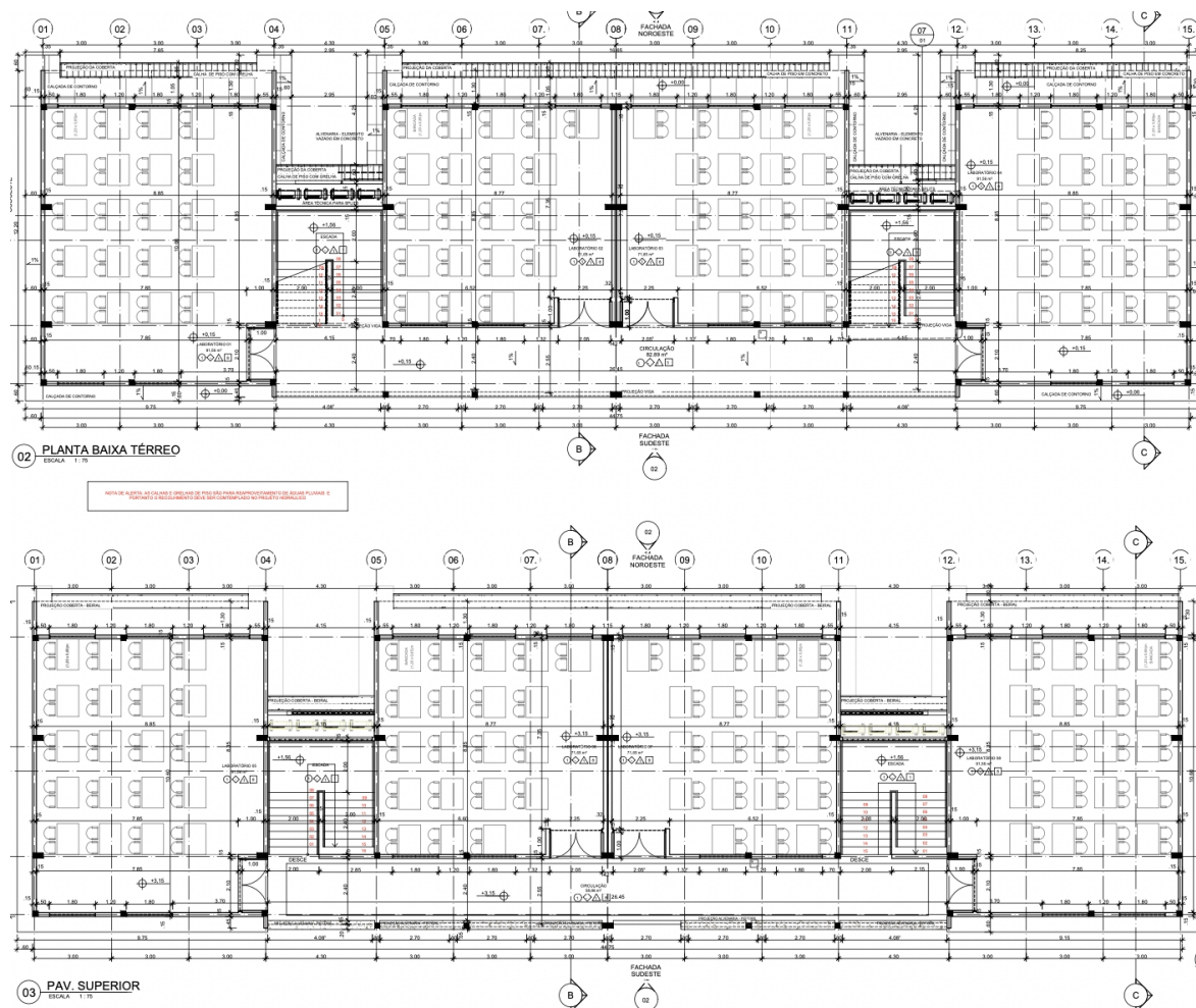
Figura 3 - Planta dos pavimentos térreo e superior dos blocos de laboratórios do campus.
